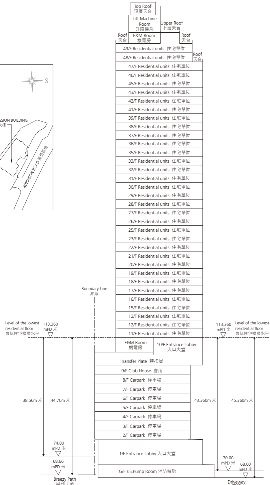
Cross-Section Plan C 橫截面圖 C
